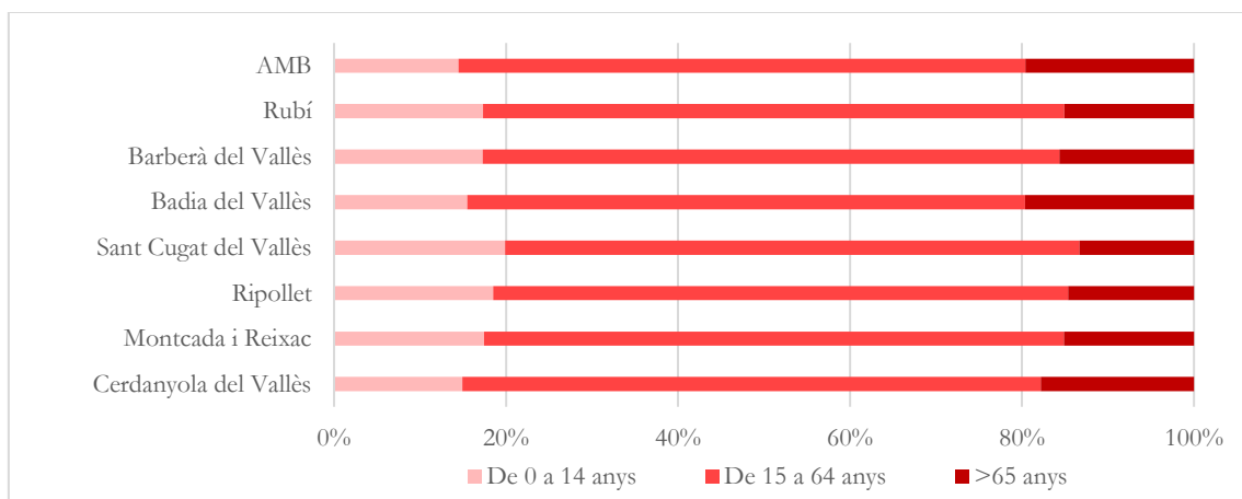
Figura 2.5. Estructura d'edats. Subàmbit metropolità i AMB, 2017.
