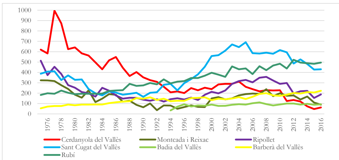
Figura 2.9. Creixement natural 1 . Subàmbit metropolità, 1976-2017.
